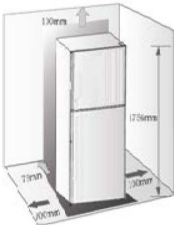
Малюнок-схема рекомендованого розміщення холодильного приладу
