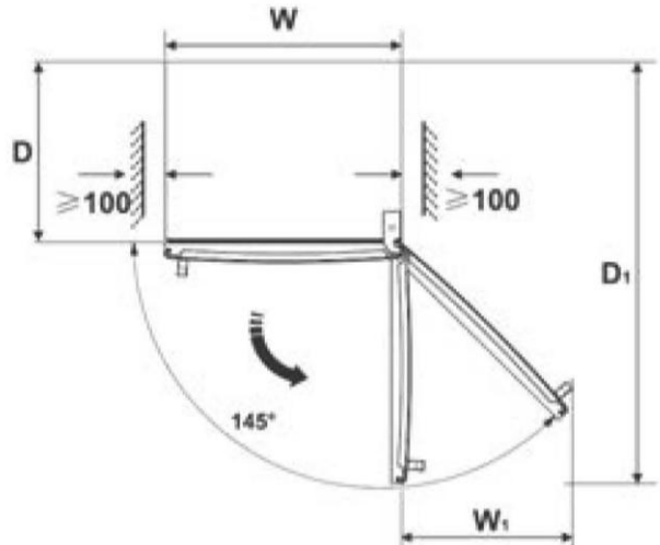
Малюнок-схема рекомендованого розміщення холодильного приладу
