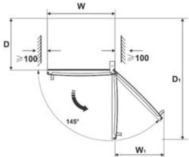
Рисунок-схема рекомендуемого размещения холодильного прибора
